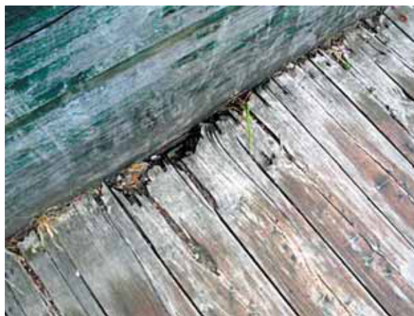
Figure 42 - Zone de mauvaise ventilation entraînant la dégradation du bois.
