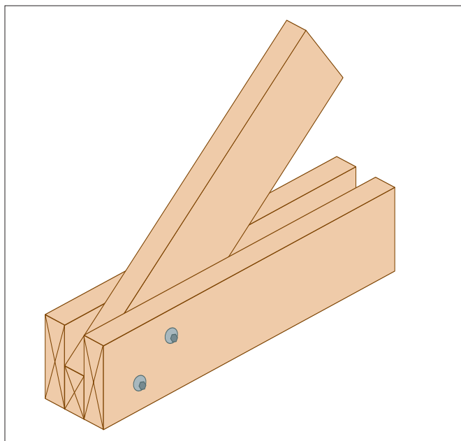
Figure 6 - Assemblage boulonné.
